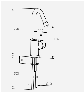
Tvättställsblandare MA-nr 70 28 05 RSK-nr 822 00 66 MA-nr 70 28 06 RSK-nr 822 00 68* */ med lyftventil
