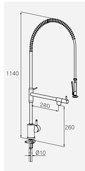
Köksblandare Mora Izzy Profi MA 70 28 40 RSK-nr 830 40 11
