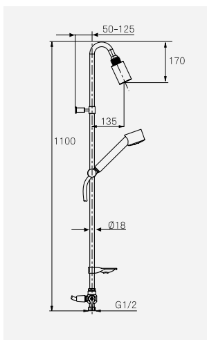
Takdusch med handdusch MA 130283 RSK-nr 893 21 58
