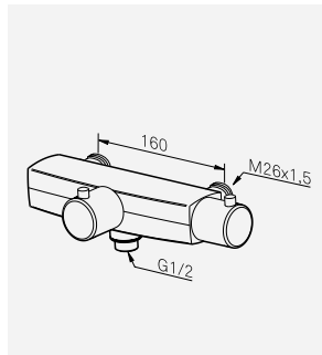
Duschblandare MA 15 08 10 RSK-nr 834 39 60 MA 15 08 15 RSK-nr 834 39 61* */ duschuttag uppåt
