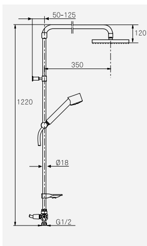
Takdusch med handdusch MA 130289 RSK-nr 893 21 63
