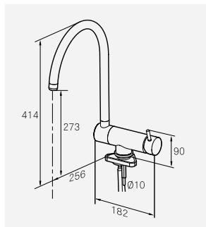
Köksblandare Mora Izzy Turnie med fällbar pip MA 70 30 46 RSK-nr 831 82 21
