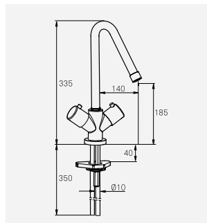
Köksblandare MA 70 28 10 RSK-nr 830 40 04
