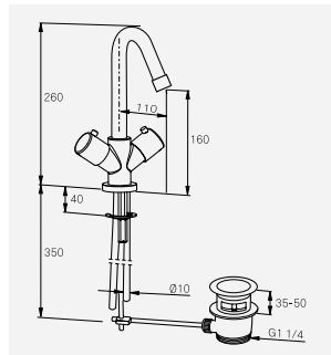
Tvättställsblandare MA-nr 70 28 16 RSK-nr 822 00 50 MA-nr 70 28 15 RSK-nr 822 00 49* */ utan lyftventil
