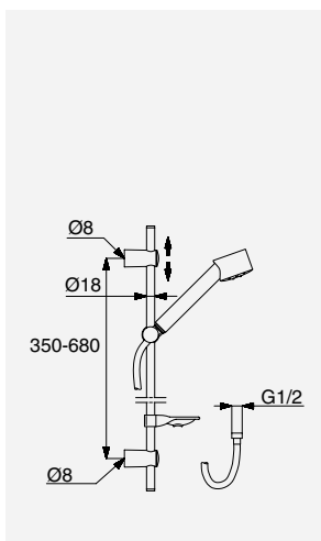
Duschset MA 130167 RSK-nr 893 21 55
