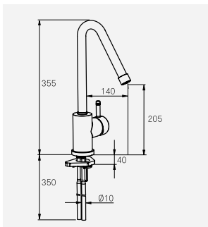
Köksblandare MA 70 28 00 RSK-nr 830 40 09
